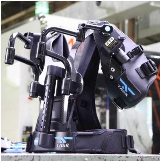
▲アシストスーツ『TASK AR1.0』
